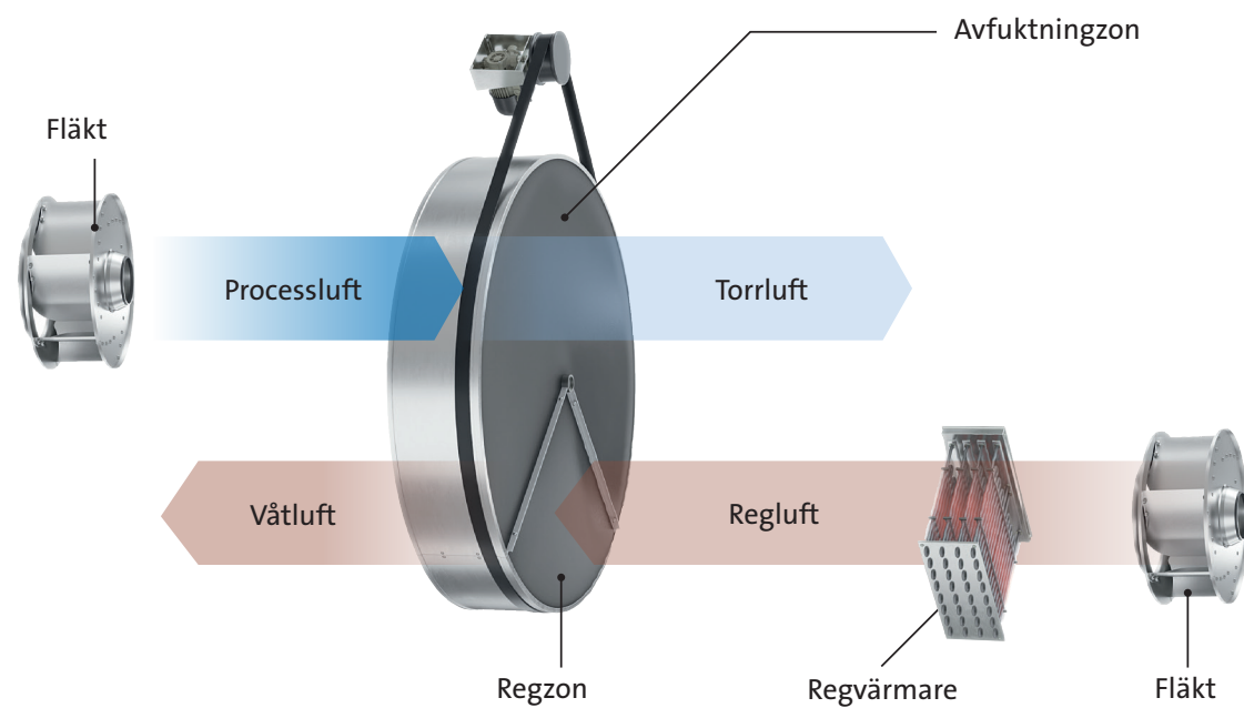
Figur 2: Funktionsprincip för en sorptionsavfuktare
