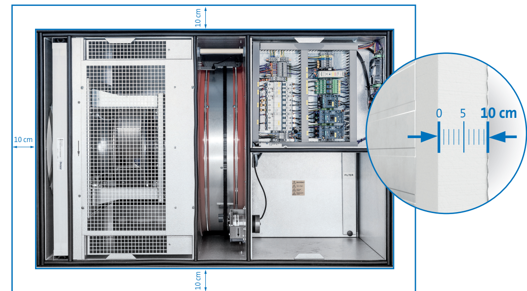
Figur 4: Avfuktare med 100 mm isolering för användning utanför fryslager
